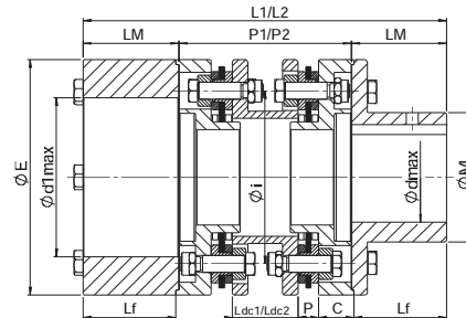
DCAMPMG
