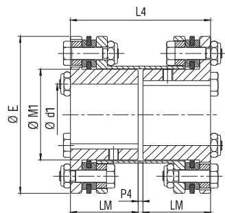
Ausführung DC2MR
