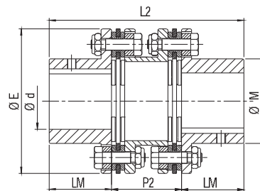
Ausführung DCC
