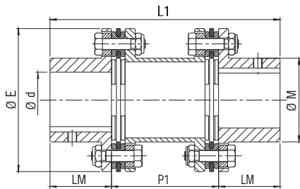
Ausführung DCL
