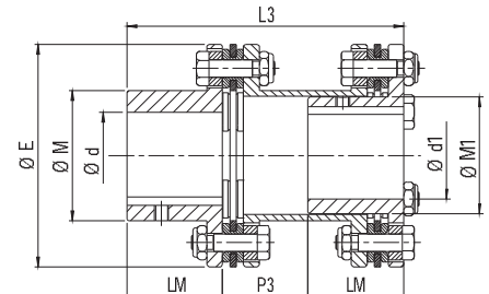
Ausführung DC1MR
