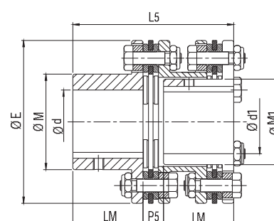
Ausführung DCC1MR
